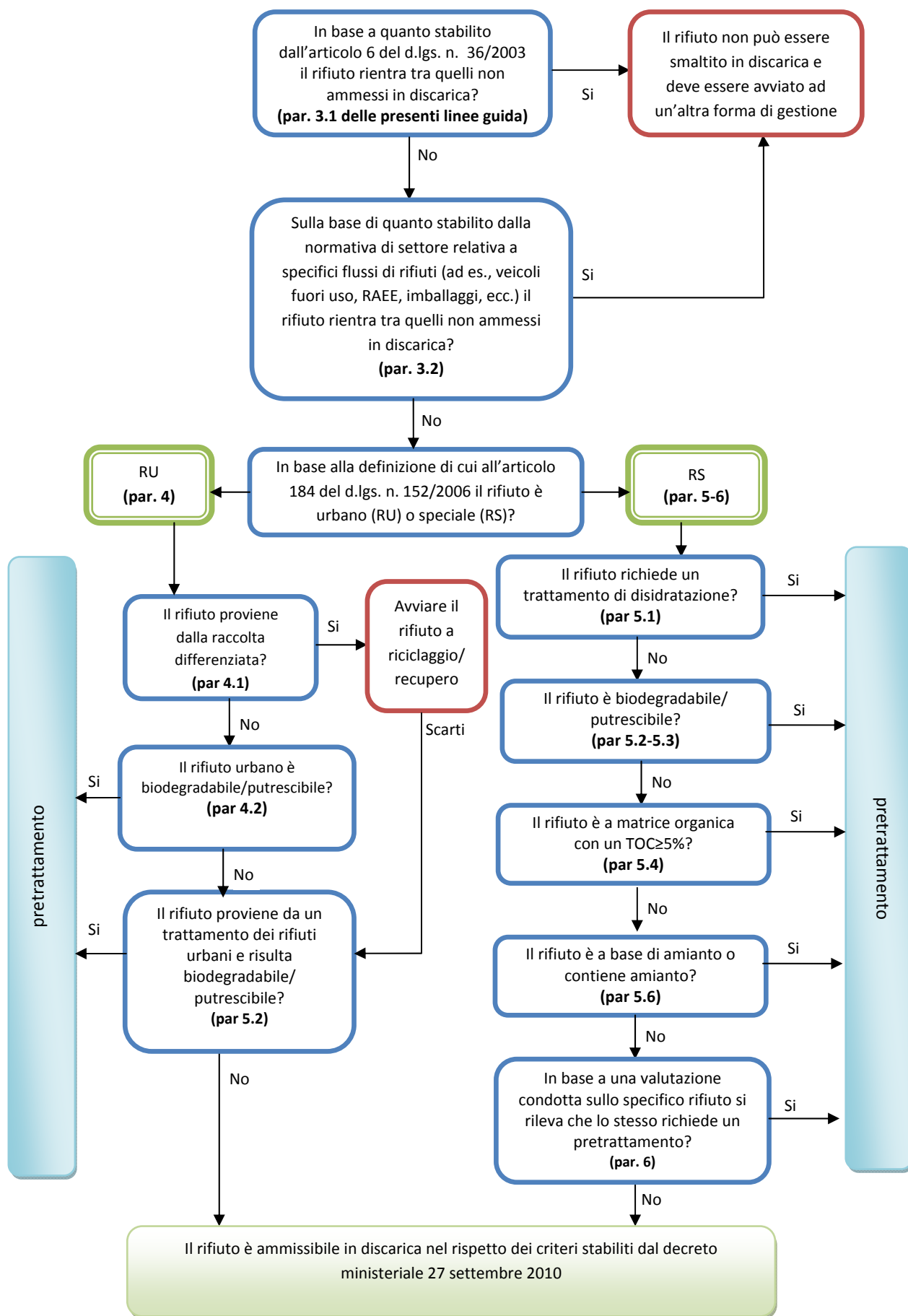
Figura 1 - Schema decisionale
